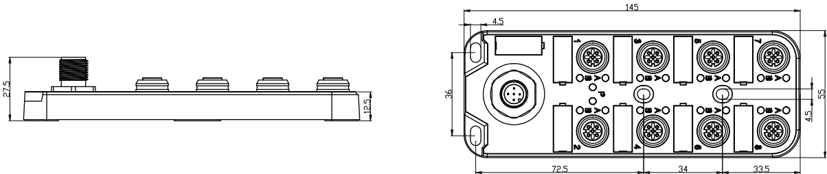
信号接口图
