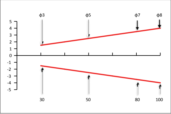
OSQ18-AK50/100 光斑图 单位 (mm)
