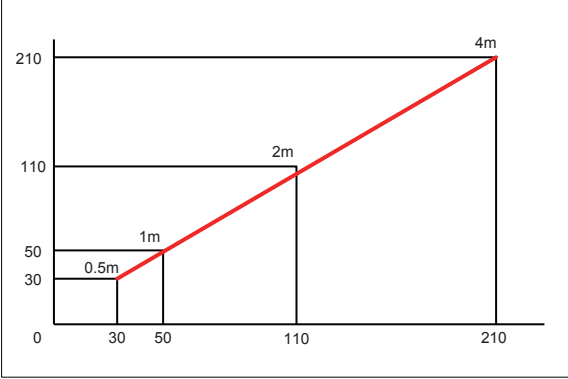
OSQ18-RP/R 光斑图 单位 (mm)
