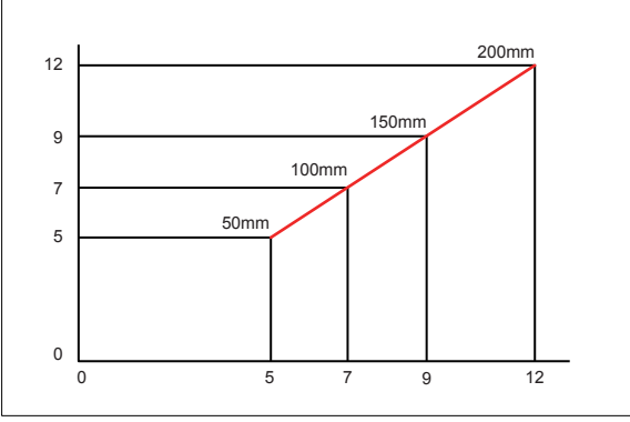
OSQ18-AK150/200 光斑图 单位 (mm)
