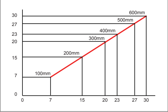
OSQ18-K 光斑图 单位 (mm)
