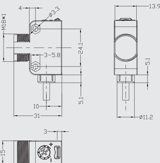
2m线缆
