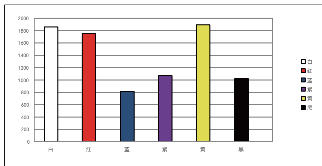
OS50-K1000VR5漫反衰减图
