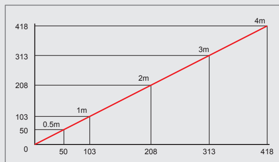
OS50-K7000 光斑图 (cm)
